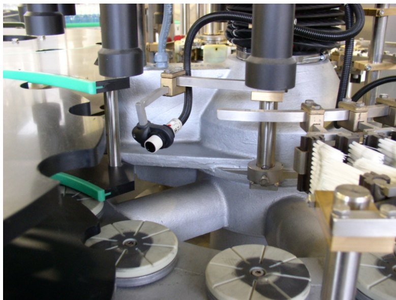
Snímač etikety v etiketovačce Gernepe - PEPSICO, Toma Teplice nad Metují, Česká Republika
